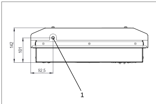
Illustration 13 – Raccordement de l'évacuation du condensat PWI
