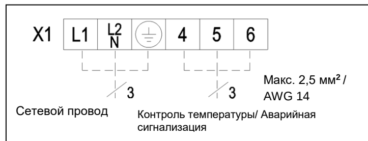
Рис. 15 – Электрическое подключение
