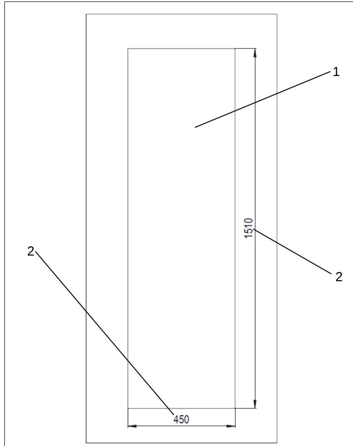
Рис. 8 - Внешний вид распределительного шкафа Вырез для воздухо-водяного теплообменника PWI
