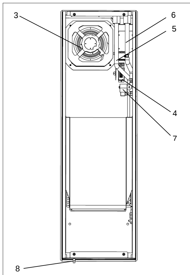
Illustration 2 – Vue intérieure Échangeur thermique air/eau
