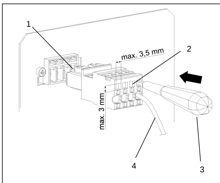
Immagine 16 - Connessione dello scambiatore di calore aria/acqua
