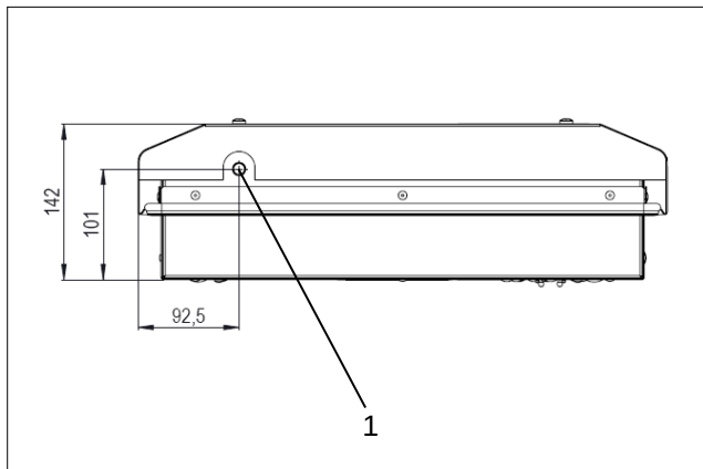
Рис. 14 – Подключение отвода конденсата PWI
