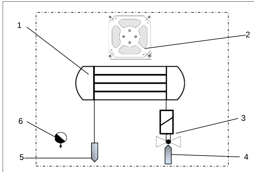
Рис. 3 - Холодильный контур
