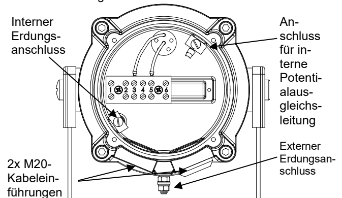
Abb. 4 Deckel Innenansicht
