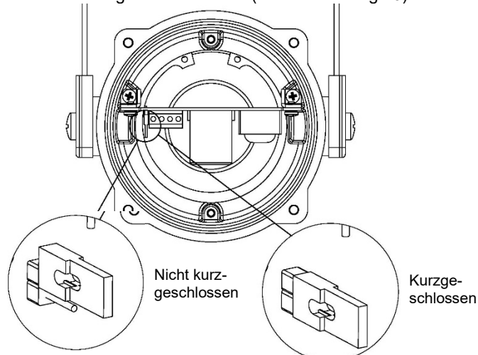
Abb. 6 Steckbrückenkonfiguration
